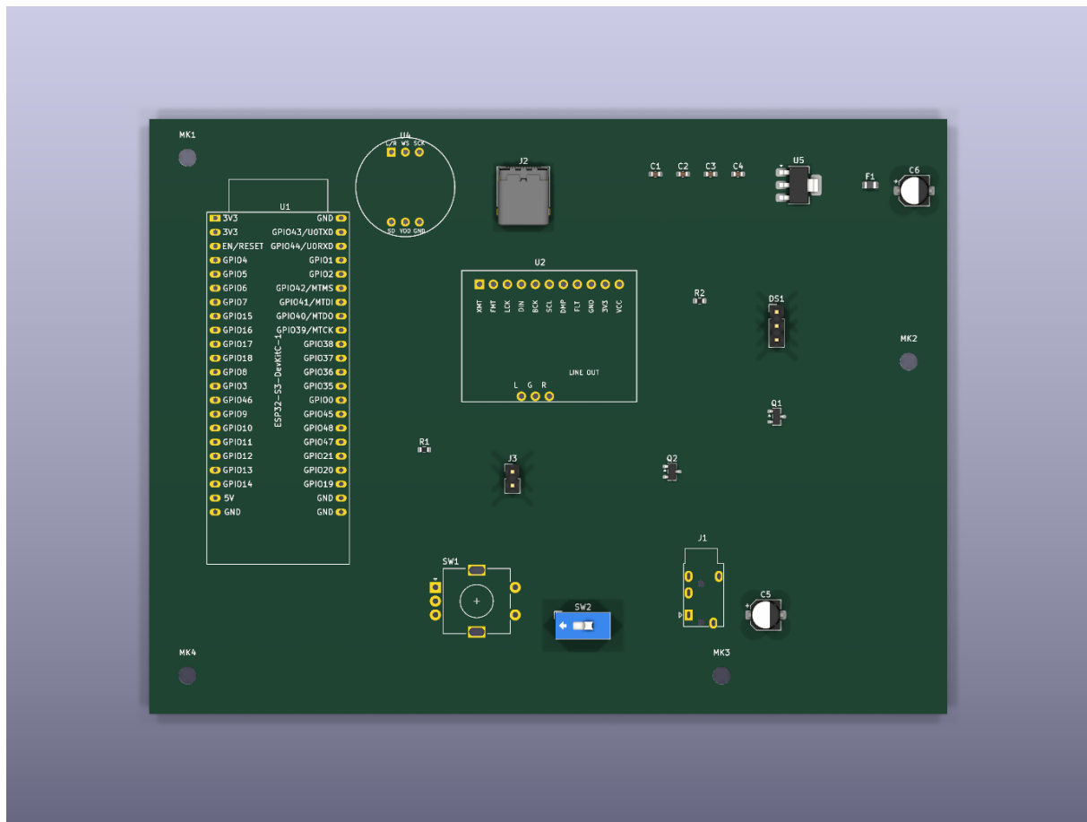
Fig. 2 - Implantation du PCB (rendu KiCad) : placement des composants, footprints reels et trous M3.
