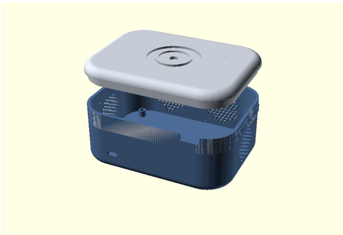
Fig. 6 - Vue éclatée du boîtier v6 : capot a molette + bac (4 HP actifs : 2 facade + 2 bouts).
